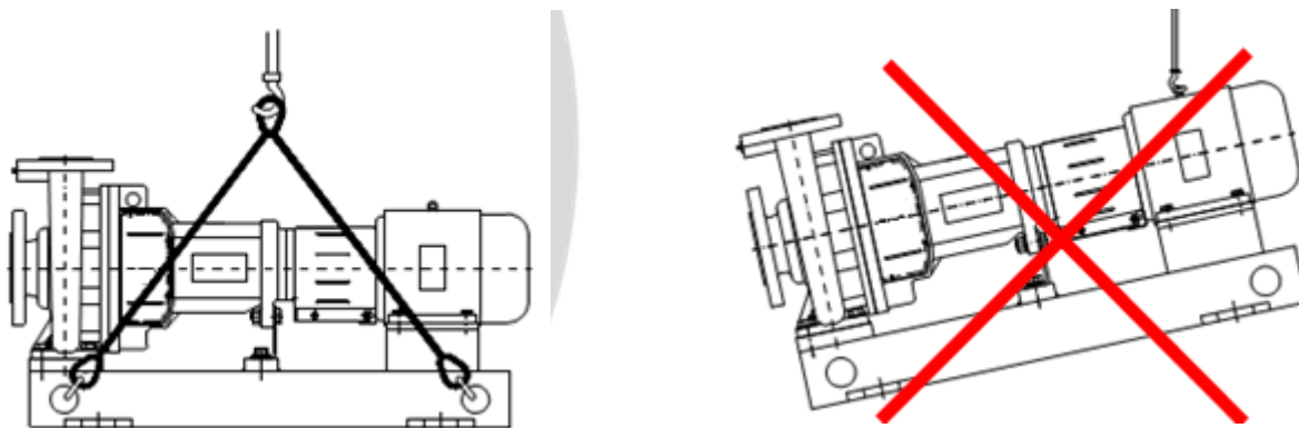
Рисунок 1 Схема строповки агрегата электронасосного серии SMA(C)
